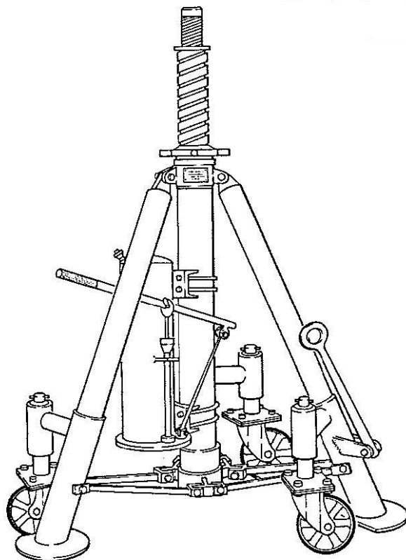
固定高型三脚型ジャッキ仕様
